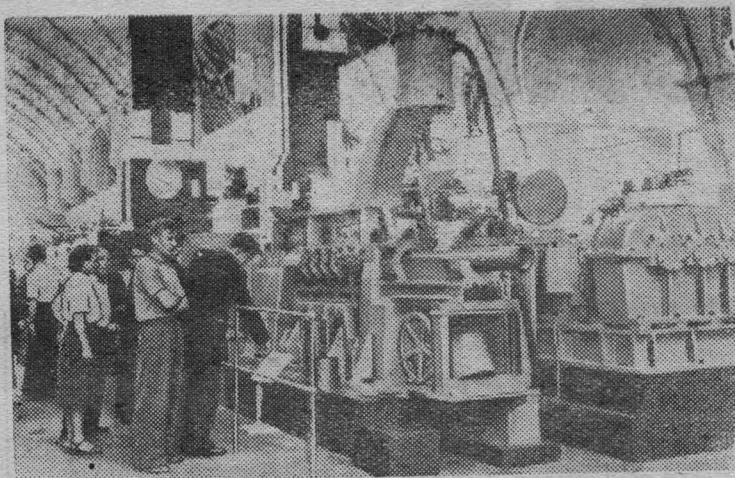
Москва. Всесоюзная промышленная выставка 1956 года. На снимке: посетители в павильоне «Машиностроение» осматривают стан для спиральной сварки труб.
