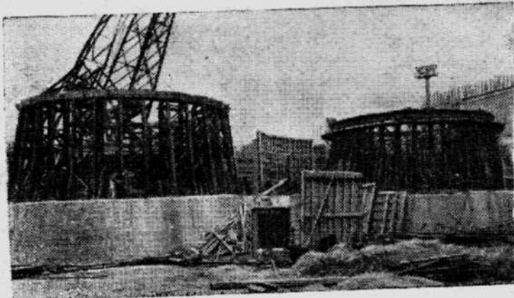
Горьковская область. В конце этого года на Горьковской гидроэлектростанции должна быть пущена в эксплуатацию первая турбина.
