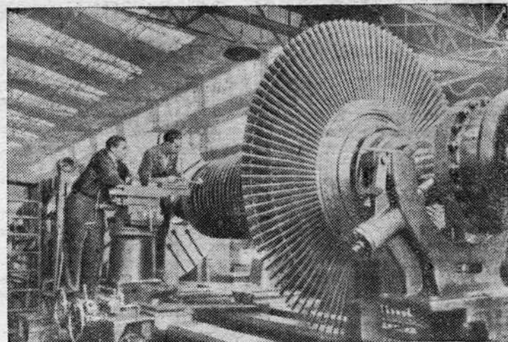
Ленинград. Коллектив паротурбинного цеха металлического завода имени Сталина изготовил турбину высокого давления мощностью 50 тысяч киловатт.
