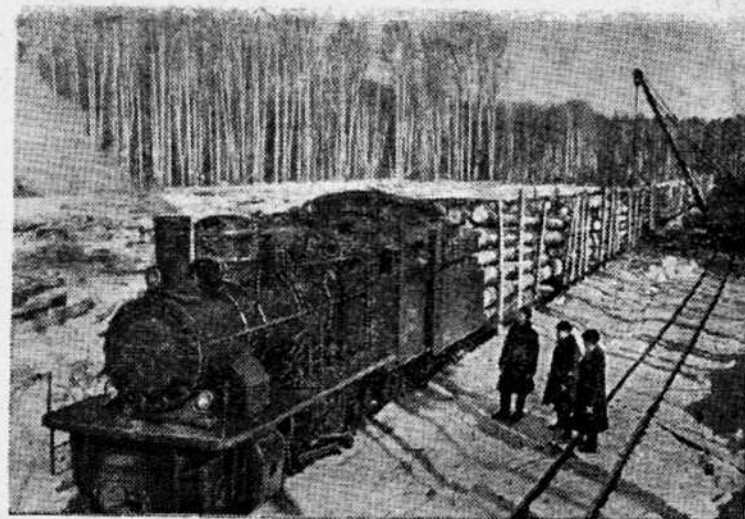
Томская область. Работая по циклическому методу, коллектив мастерского участка старшего мастера Я. П. Рымши Тимирязевского леспромхоза вдвое увеличил среднесуточную заготовку леса, трелевку и погрузку его на железнодорожные платформы. Этому участку присуждено переходящее Красное знамя Министерства лесной и бумажной промышленности СССР и ВЦСПС.
