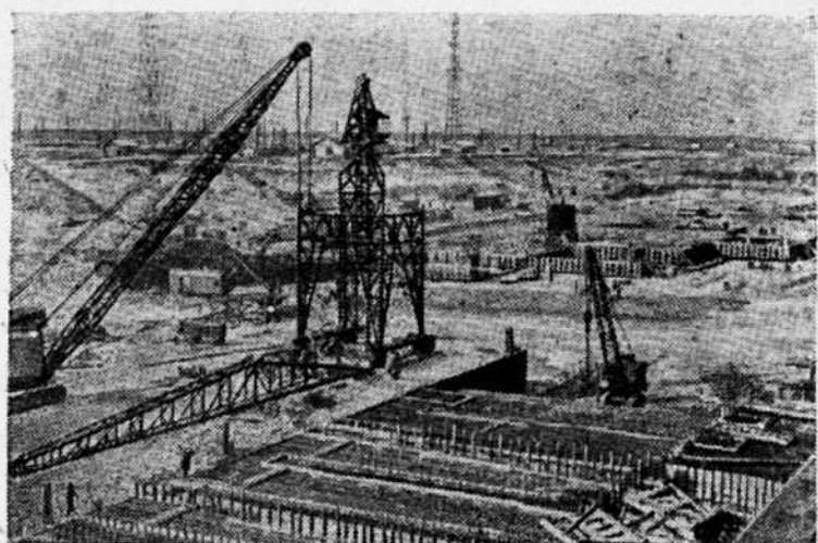
На строительстве Каховской ГЭС. Соревнуясь в честь 300-летия воссоединения Украины с Россией, коллектив строителей обязался построить Каховскую ГЭС на год раньше установленного срока. Это обязательство успешно выполняется.
