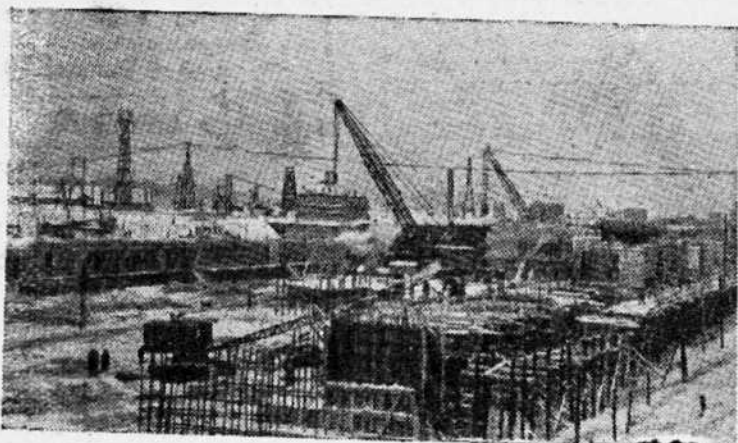
На реке Каме, близ города Молотова, сооружается Камская ГЭС, которая в этой пятилетке должна войти в строй и дать мощное подкрепление энергетической базе Урала. Для Камской ГЭС не будет строиться специальное здание — она разместится в теле водосливной плотины. Шлюз будет разделен на два канала. Через один из них будут пропускаться плоты с лесом. Второй канал предназначен для судоходства.
