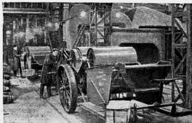
Рязань. Завод «Рязсельмаш» наладил серийный выпуск картофелеуборочных комбайнов «КОК-2». На полях, где картофель посажен четырехрядными картофелепосадочными машинами, комбайн выкапывает клубни, отделяет их от земли и ботвы и сыплет в тару. За один проход машина убирает два ряда картофеля. Комбайн в пять раз сокращает затраты труда по сравнению с конно-ручной уборкой.
