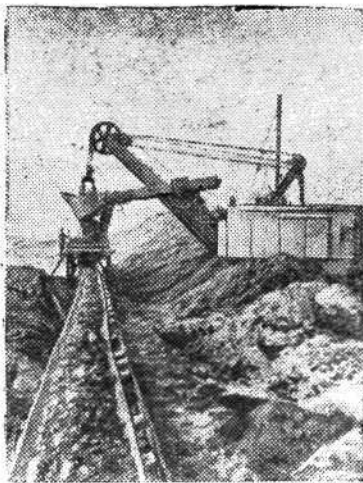
Иркутская область. Храмцовский разрез № 1, в котором добыча производится открытым способом, в 1953 году дал стране сверх плана десятки тысяч тонн угля.
