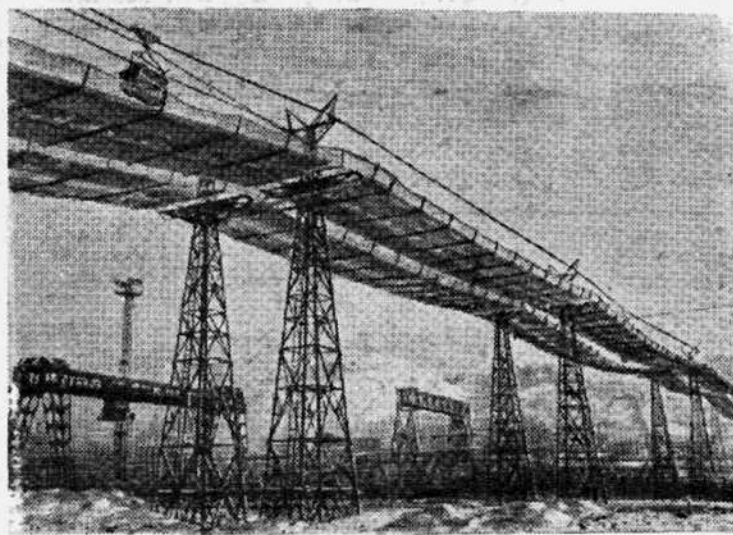
Куйбышевгидрострой. Вступил в строй участок канатной подвесной дороги от камнедробильного завода на горе Могутовой до бетонного завода. На этом участке по четырем стальным канатам движется более 70 вагонов, которые перевозят 180 тонн щебня в час. На снимке: участок канатной подвесной дороги.
