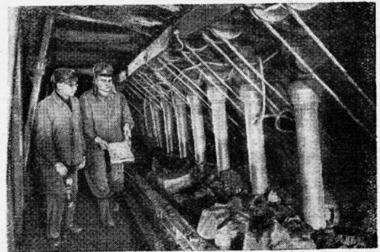
Тула. На шахте № 12 треста «Щекинуголь» испытывается новый металлический передвижной щит Ш-52 длиной 50 метров. Он предназначен для механизированного крепления горных выработок. Внедрение этого щита создаст условия для осуществления комплексной механизации всех процессов угледобычи, увеличивает производительность труда, значительно снижает себестоимость и повышает безопасность работы в лаге.
