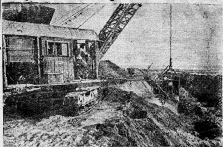
Казахская ССР. Началось строительство самостоятельного Арысь-Туркестанского канала, который явится крупнейшим ирригационным сооружением Казахстана. Канал протяженностью в 195 километров орошит свыше 117 тысяч гектаров степи. Орошаемые земли будут использованы под хлопковые плантации, посев зерновых культур и трав.
