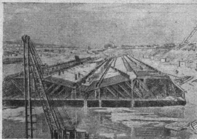
Куйбышевгидрострой. На строительстве камер нижнего судоходного шлюза идет монтаж металлоконструкций и укладка бетона.
