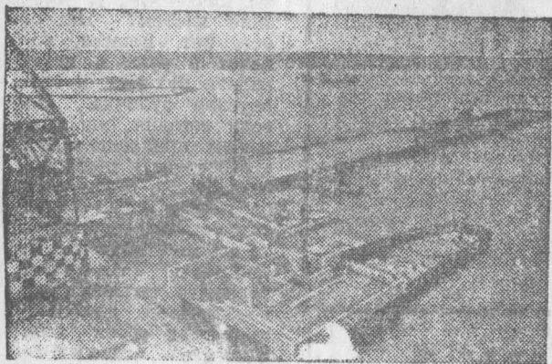
Литовская ССР. На строительстве международной переправы СССР — ГДР в Клайпеде завершены очередные этапы работ — возведены металлические конструкции двухсотметрового причального пирса. Для этого потребовалось вбить в морское дно 2700 тонн металлических свай. Сейчас ведутся работы по укладке грунта на всей площади причала, на которой затем будут монтироваться массивные железобетонные плиты.
