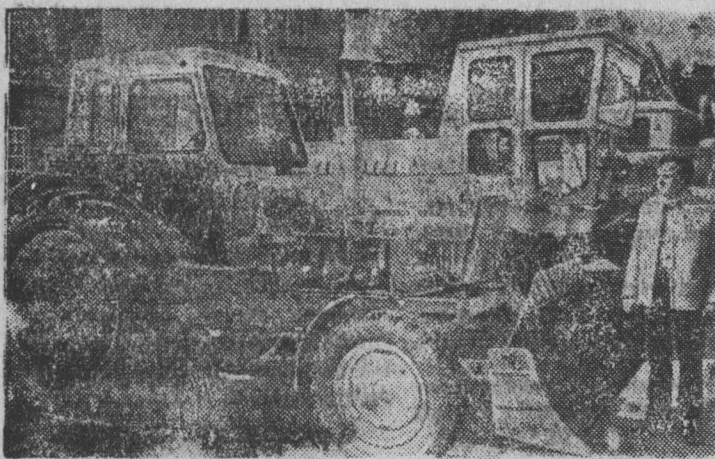
Москва. На ВДНХ СССР в разделе «Строительство» (на Фрунзенской набережной) демонстрируются новые дорожные и строительные машины научно-производственного объединения «Дормаш». Министростроймаш экспонирует бульдозер ДЗ-102, установленный на тракторе МТЗ-80/82. Агрегат используется при разработке грунта, при планировке площадок и грунтовых дорог, для очистки их от снега. Производительность агрегата при перемещении грунта на расстояние 30 метров — 55—60 кубических метров в час. Новый бульдозер намечен к серийному выпуску в 1977 году. НА СНИМКЕ: бульдозер ДС-102.
