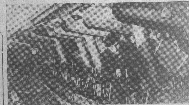
ТУЛЬСКАЯ ОБЛАСТЬ. Строительство подземного гиганта «ОКП» — самого крупного в нашей стране механизированного комплекса для выемки угля — завершено в цехах Угловского машиностроительного завода. Комплекс будет действовать в ломах длиной 120 метров и предназначен для механизации и автоматизации основных и вспомогательных работ в очистном забое.
