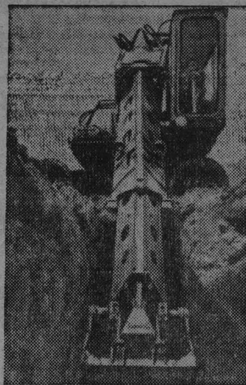
ЧЕХОСЛОВАКИЯ. Универсальный кран «Сатурн-035» для строительства дорог создан на машиностроительном заводе Детва в Центральной Словакии. Новый агрегат может быть использован как грейфер и канавокопатель.
