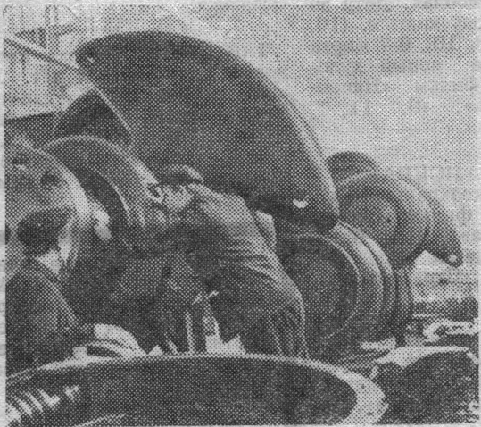
На снимке: дизелисты А. Сенченков (слева) и В. Удалой проверяют коленчатый вал корабельного дизеля в новом цехе Брянского машиностроительного завода. Этого цеха два года назад еще не было на предприятии. Фото В. Кунова. Фотохроника ТАСС.
