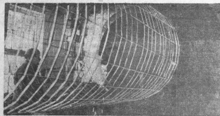
Московский завод железобетонных изделий № 15 выпускает трубы диаметром от 300 до 1200 миллиметров. Они находят широкое применение в народном хозяйстве.
