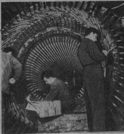
Завод электрооборудования во Вроцлаве — основной поставщик генераторов для польских электростанций. На снимке: сборка турбогенератора с водородным охлаждением. Фото ЦАФ — ТАСС.
