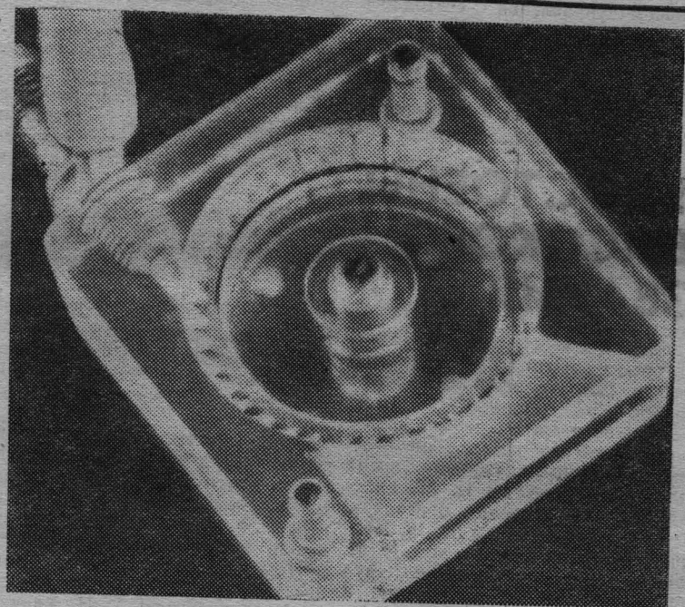
Модель «холодной» турбины из органического стекла. Она работает на углекислом газе при комнатной температуре. Газ вырабатывают... микроорганизмы. Идею использования бактерий для выработки углекислого газа предложил московский изобретатель А. Г. Пресняков. Осуществить ее помогли работники Всесоюзного научно-исследовательского института новых строительных материалов.
