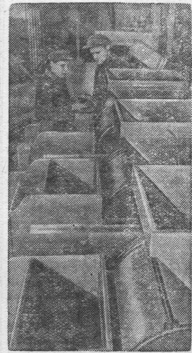
Киевский завод мельничных машин им. Дзержинского начал изготавливать машины для переработки проса — просорушки. На снимке: В слесарно-сборочном цехе завода. Мастер цеха А. И. Натоптанный и контрольный мастер В. Г. Розов осматривают готовые просорушки.
