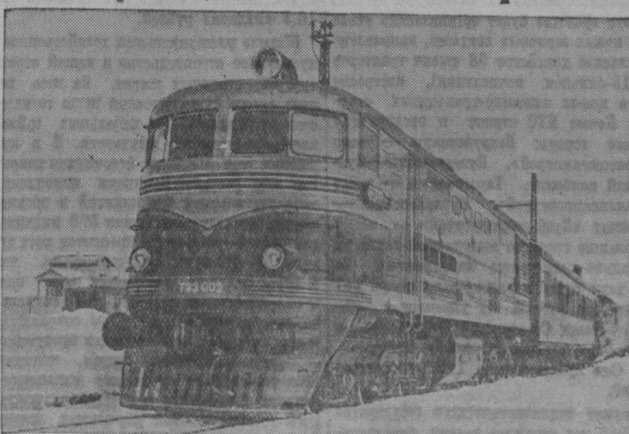
Под Москвой проводится испытание опытного тепловоза «ТЭ-3». Новый тепловоз способен водить товарные составы со скоростью до ста километров в час. Предусмотрена возможность значительного повышения скорости для тепловозов в пассажирском варианте. Мощность двух секций тепловоза «ТЭ-3» — 4.000 лошадиных сил.
