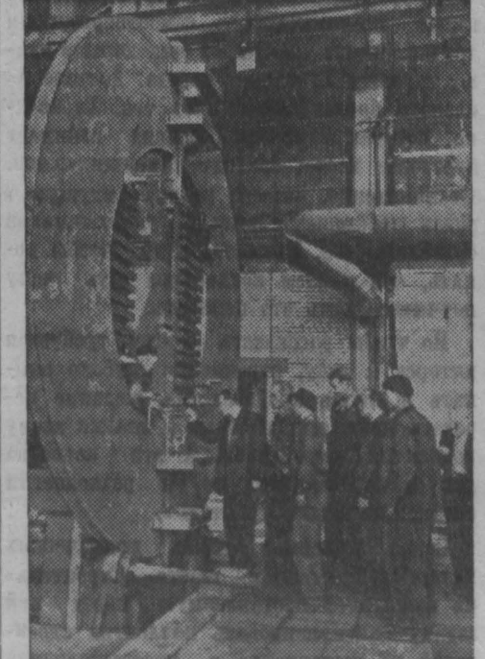
Ленинград. Коллектив института электросварки имени академика Патона Академии наук Украинской ССР много работает в области автоматизации электросварочных работ. Им создан малогабаритный вертикально-электросварочный сварочный аппарат, предназначенный для сварки дисков и других деталей толщиной от 60 до 250 миллиметров. Для того, чтобы использовать аппарат в одном из цехов завода «Электросила» имени С. М. Кирова смонтирована специальная установка. С вводом в эксплуатацию нового сварочного аппарата производительность увеличится в несколько раз.
