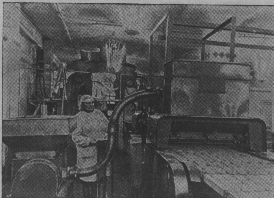
На Ленинградском мясокомбинате имени С. М. Кирова пущена в эксплуатацию новая механизированная линия для приготовления котлет. Поточная линия состоит из фаршеприготовительного агрегата непрерывного действия, котлетного автомата, конвейера для укладки котлет, транспортных лент, подающих тару и отправляющих уложенные котлеты в экспедицию. За смену на механизированной поточной линии изготовляется до 500 тысяч штук котлет. На снимке: автоматизированная линия для производства котлет. (Фотохроника ТАСС).
