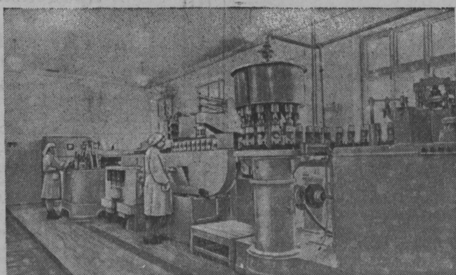
Ленинградским машиностроительным заводом «Красная вагранка» изготовлен автомат для производства бумажных бутылок и расфасовки в них молока. Он склеивает из тонкого бумажного картона молочные бутылки, парафинирует, охлаждает их, наполняет молоком и укупоривает. Производительность автомата — 2,5—3 тысячи бутылок в час. На снимке: автомат для изготовления бумажных бутылок и разливки молока. Фото Э. Евзерихина. (Фотохроника ТАСС).
