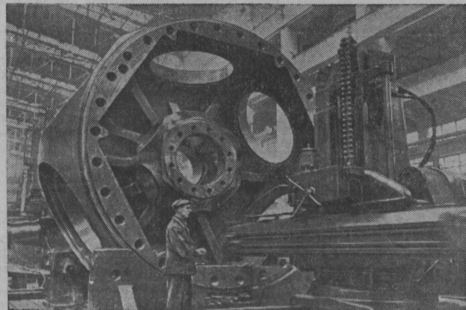
Ленинград. Новыми победами в труде отмечают дни подготовки к празднованию 37-й годовщины Октябрьской революции завод имени Сталина. Включившись в шестой куйбышевской турбины и успешно его выполнили. На снимке: в гидротурбинном цехе. Строгальщик А. Ф. Шалаев за обработкой втулки рабочего колеса шестой куйбышевской турбины. Фото А. Михайлова.
