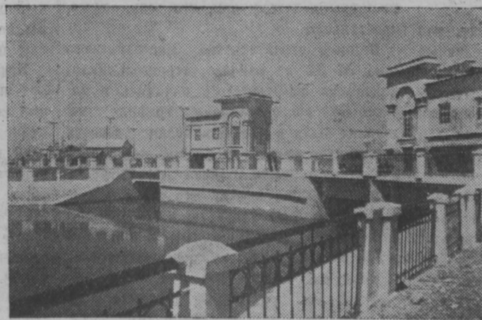
Ставропольский край. Мощные железобетонные устройства главного шлюза Кубань—Егорлыкской оросительной системы направляют кубанскую воду по 54-километровому каналу в засушливые районы края.
