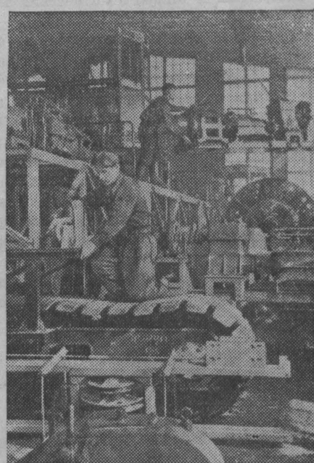
Ивановский завод «Исторфмаш» освоил выпуск модернизированных оборочно-перевалочных машин марки «УПФ-2». Эта машина служит для уборки фрезерного торфа методом перекачки. Производительность «УПФ-2» — 720 кубометров в час. Она обслуживается двумя работниками—машинистом и его помощником и заменяет труд 300 рабочих. На снимке: на переднем плане бригадир слесарей Н. М. Мельников за сборкой машины марки «УПФ-2». Фото Ф. Карышева. (Фотохроника ТАСС).
