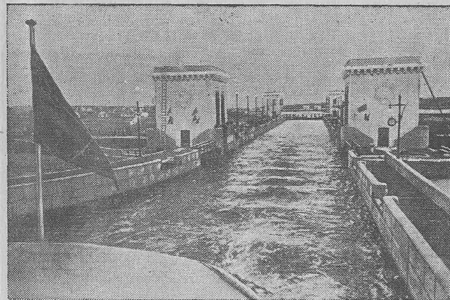
Волго-Донской судоходный канал имени В. И. Ленина. На снимке: шлюз № 8 со стороны верхнего подхода. Фото В. Егрова.
