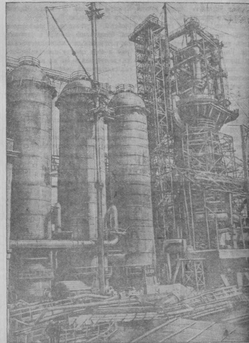
На снимке: на строительстве новой домы № 4 «Азовстали» (Мариуполь). Фотохроника.
