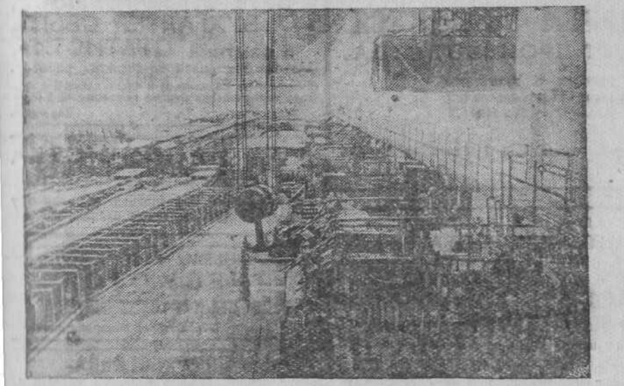
16 июля вступил в строй новый мощный прокатный стан «350» на Макиевском металлургическом заводе им. Кирова. На снимке: общий вид зала прокатного стана «350».
