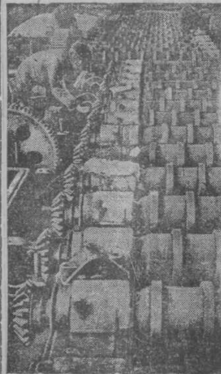
Краматорский машиностроительный завод им. Орджоникидзе (Донбасс) изготовил для тонколистного стана «Запорожстали» рольганг длиной 32 метра. На снимке: сборка рольганга для «Запорожстали». (Союзфото).
