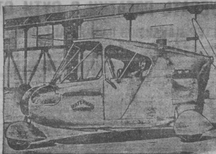
Самолет-автомобиль. Американский конструктор В. Уотермен сконструировал оригинальный самолет, который может быть после приземления и снятия крыльев использован как автомобиль. Самолет снабжен шестцилиндровым мотором «Студебекер». Скорость его в воздухе до 200 км. в час, на земле до 80 км. в час. На снимке: самолет-автомобиль после снятия с него крыльев на аэродроме в Санта-Моника (штат Калифорния). (Союзфото).
