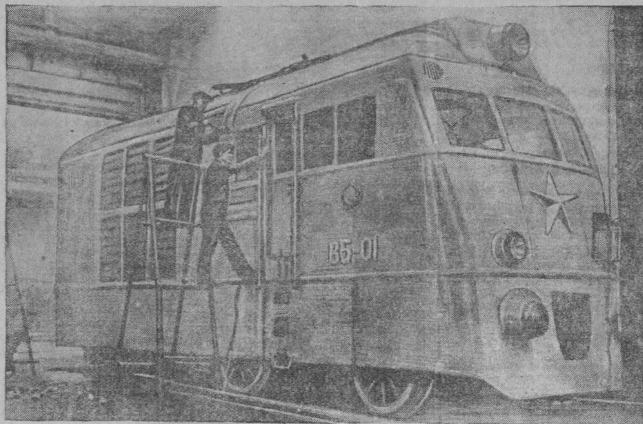
Коломенский машиностроительный завод им. В. В. Куйбышева заканчивает монтаж и сборку основных узлов опытного паровоза высокого давления, обтекаемой формы. Этот паровоз даст большую экономию топлива. На снимке: паровоз высокого давления „B5-01“. Слесари-сборщики тт. Н. И. Голубков и Н. Г. Федотов заканчивают отделку паровоза. Союзфото.
