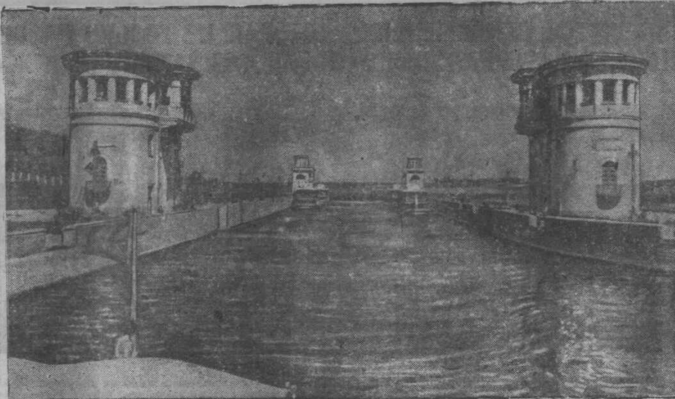
Канал Москва—Волга. На снимке: общий вид шлюзовой камеры № 5.
