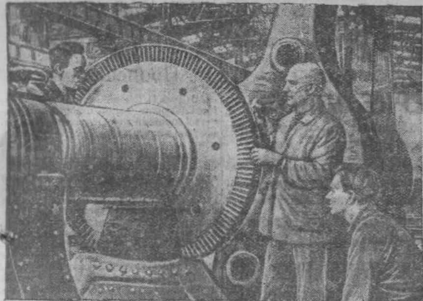
На Ленинградском заводе им. Сталина производится сборка ротора быстроходной гигантской турбины им. Серго Орджоникидзе мощностью 100 тысяч киловатт. На снимке: бригада орденосца П. Е. Хинейко за сборкой ротора турбины. Слева направо—М. П. Кузнецов, П. Е. Хинейко и М. В. Грибач. Фото Л. Зиверта (Союзфото).
