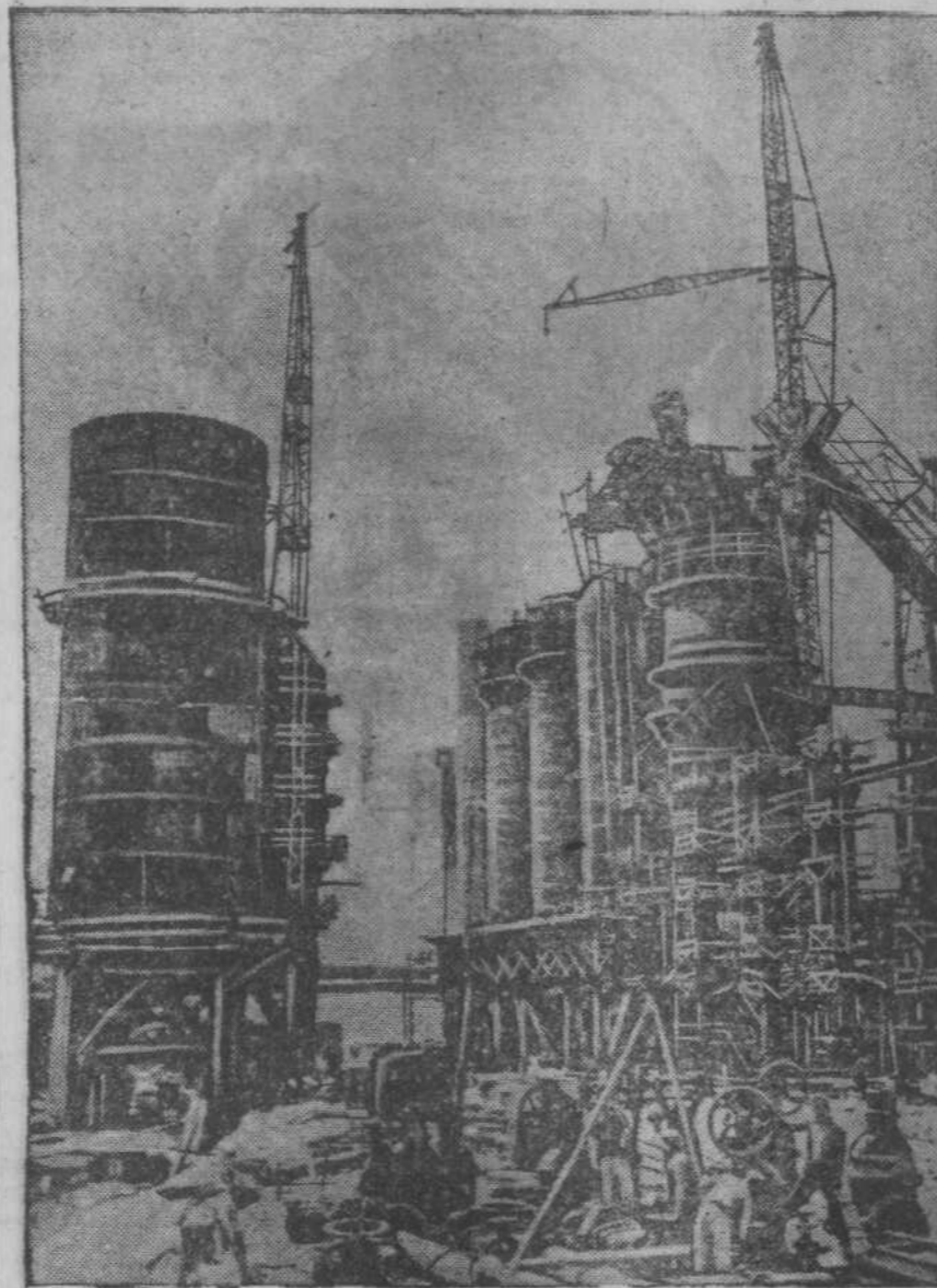
На Запорожском металлургическом заводе «Запорожстали» строится мощная доменная печь №3. На снимке: общий вид строительства домы №3 об'емом 1300 кубических метров. Фото Ф. Кислова. (Союзфото).
