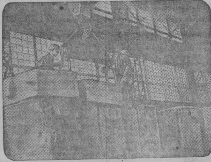
В здании изложниц стрипперного цеха. На снимке: установка утеплителей на уширенные изложницы. (Фото И. Бажина).
