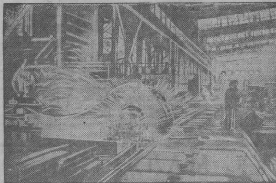
Прокатный цех. На чистовой клети стана 750 2 рельсы выходят в 60-75 метров длиной. Каждый такой рельс надо разрезать на несколько частей длиной в 12,5 метра. На снимке: пилой режут рельс.
