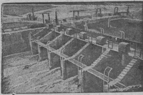
Плотина под Самаркандом. Одно из больших достижений Средней Азии к десятилетию размежевания республики
