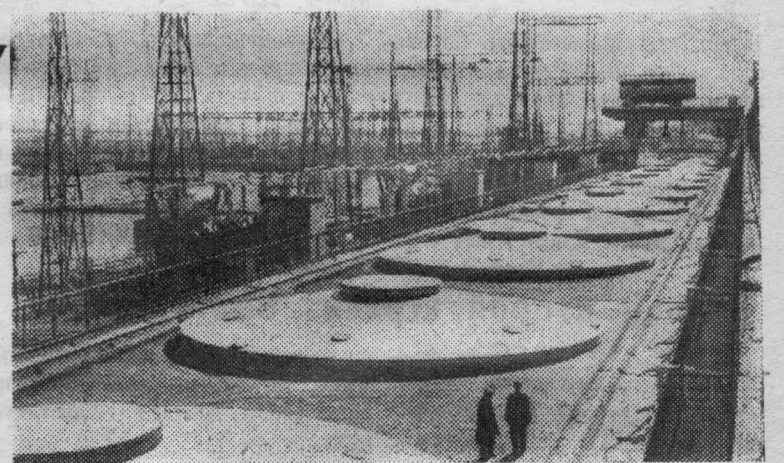
КРЕМЕНЧУГСКАЯ ГЭС. Ее мощность 625 тысяч киловатт. Это станция открытого типа, без здания машинного зала. Она уже работала более 1,5 миллиарда киловатт-часов электроэнергии. Фото Г. Верушкина. Фотохроника ТАСС.
