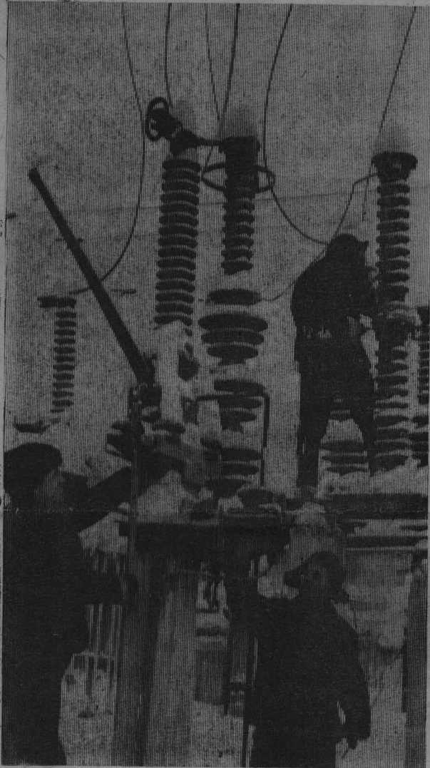
Бригада электромонтажников подстанции 110 кВ в составе В. П. Лебедева, Г. С. Курочкина и В. А. Гофмана ведет подготовку электроустановки РВС 110 кВ к включению в работу.
