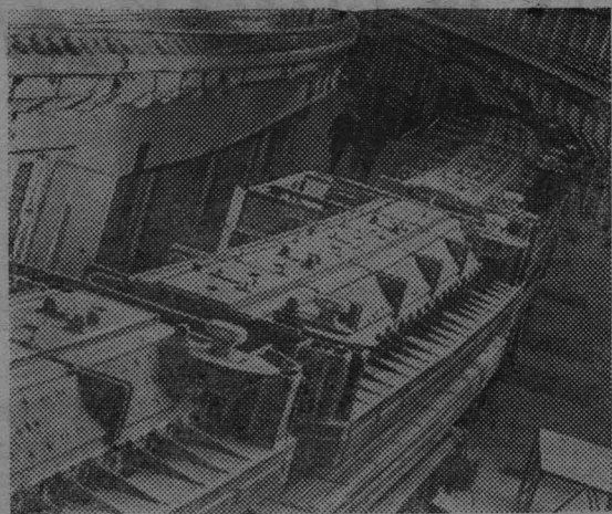
МОСКВА. Осуществлен запуск протонного синхротрона Института физики высоких энергий Государственного комитета по использованию атомной энергии СССР. Крупнейший в мире серпуховский ускоритель, на котором получен пучок протонов с энергией 70 миллиардов электронвольт, достиг проектной энергии. В процессе испытаний аппаратуры ускорителя были получены пучки протонов с энергией 76 миллиардов электронвольт, что существенно выше проектной энергии.
