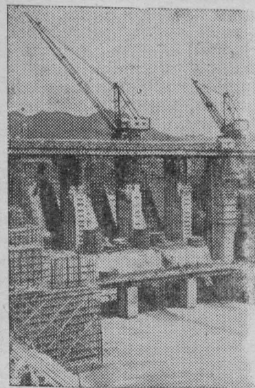
Китайская Народная Республика. На реке Синьаньцзян в провинции Чжэцзян сооружается гидроэлектростанция мощностью 650 тысяч киловатт. Созданная по проекту китайских инженеров станция даст первый ток в конце 1959 года.
