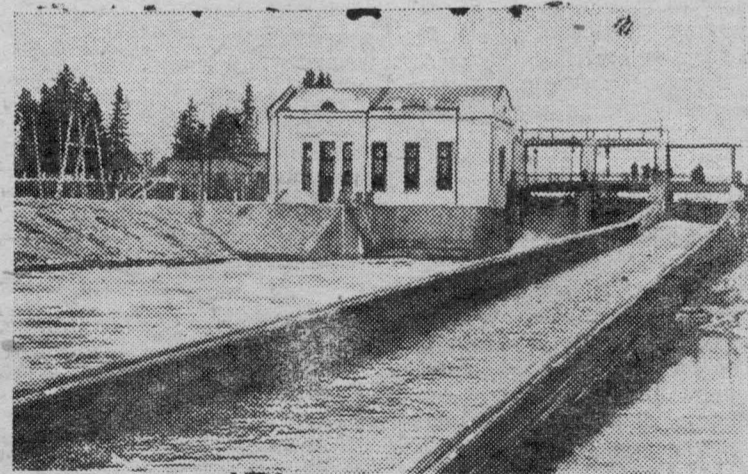
Витебская область. В Россонском районе вступил в строй первый агрегат Клястицкой сельской гидроэлектростанции на реке Ница. С пуском второй турбины мощность электростанции составит 520 киловатт. Ее энергия будет использоваться в 20 колхозах и совхозах области.
