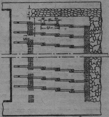
Рис. № 1. Крепление очистного забоя лавы деревом.
