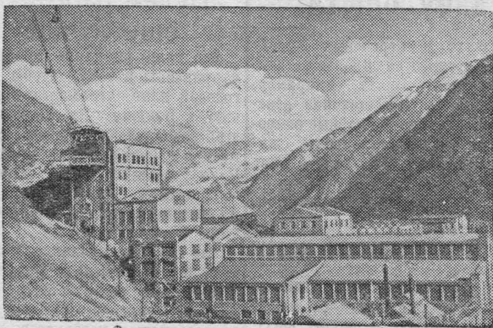
В горах Северо-Осетинской АССР за годы сталинских пятилеток построена Мизурская обогатительная фабрика по добыче цветных металлов. Общий вид Мизурской обогатительной фабрики. Фото И. Смолий.
