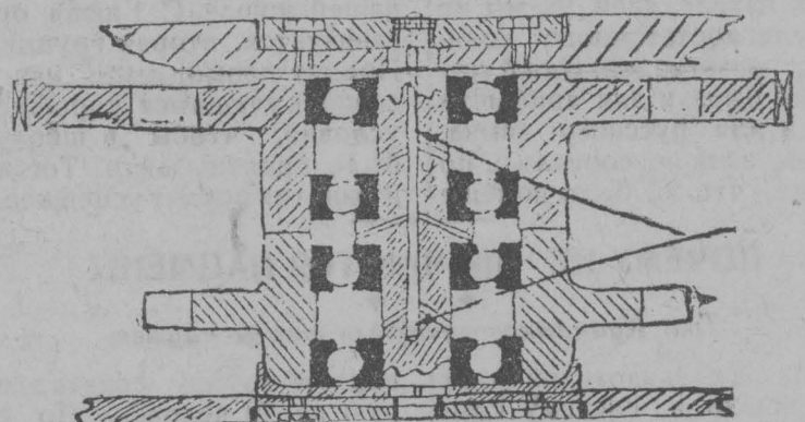
На чертеже стрелками указаны отверстия для промывки и смазки подшипников 6215
