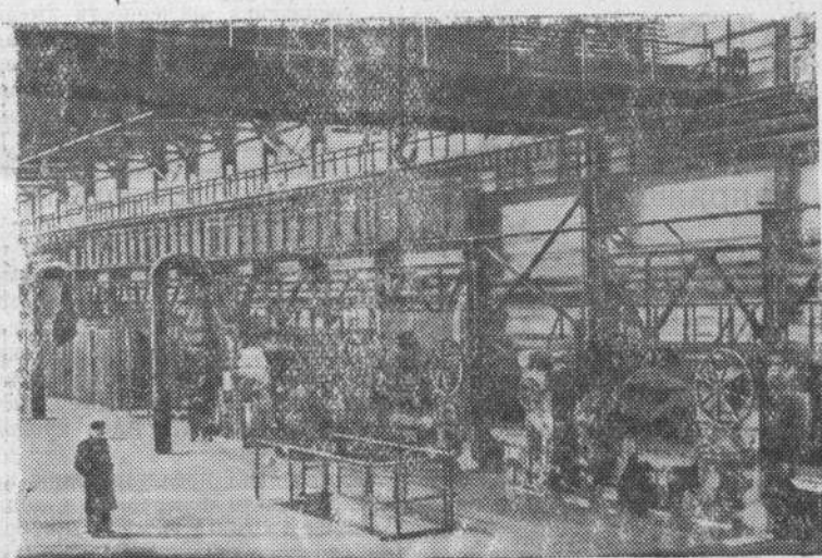
На Челябинском металлургическом заводе закончилось строительство нового прокатного стана «300». Он будет выпускать в основном прокат мелкого профиля и арматурное железо. Стан построен по последнему слову техники. Управление его узлами полностью механизировано и автоматизировано. В отличие от других в новом стане имеется одна большая нагревательная печь вместо двух малых.
