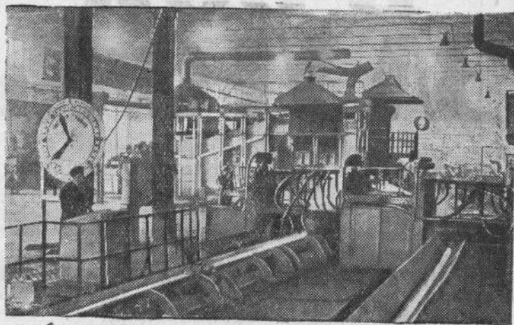
Узбекская ССР. Завод «Ташкенткабель» с начала года изготовил кабеля и провода на 30 процентов больше, чем за такой же период прошлого года. На предприятии успешно внедряется новая техника. Установлен более совершенный прокатный стан. Процесс изготовления катанки из медных слитков ведется автоматически.
