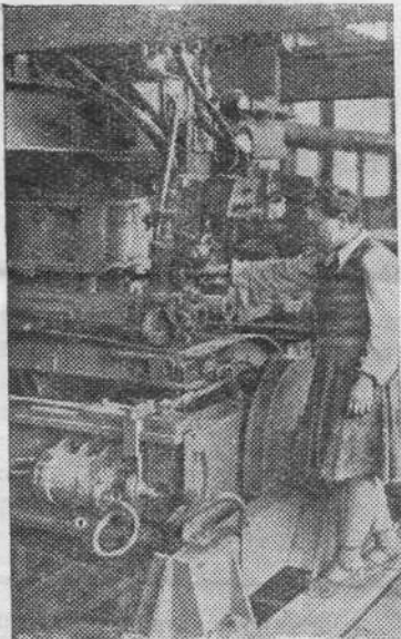
Вальцесварочный станок листа к лобовым. Приварка производится двумя автоматическими электросварочными головками под слоем флюса.
