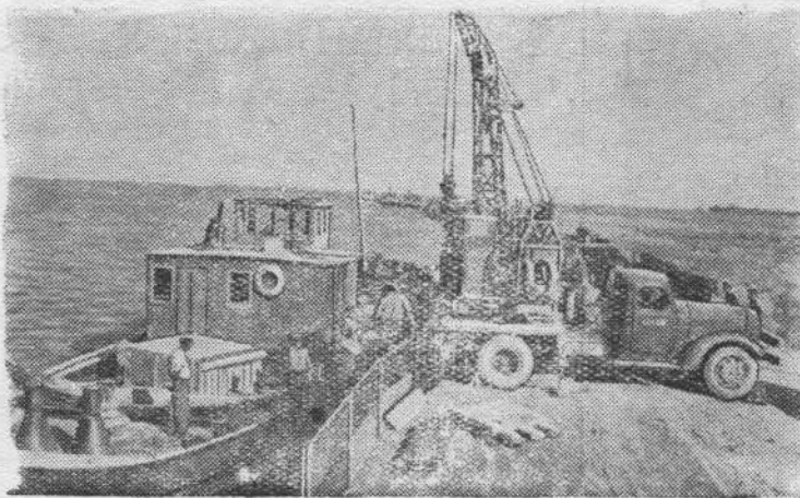
Туркменская ССР. На строительстве Кара-Кумского канала. На снимке: разгрузка с барж автокраном механизмов и строительных материалов, прибывших для строительства канала. Фотохроника ТАСС.
